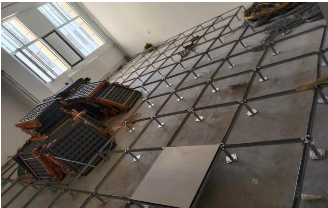
防静电地板安装
