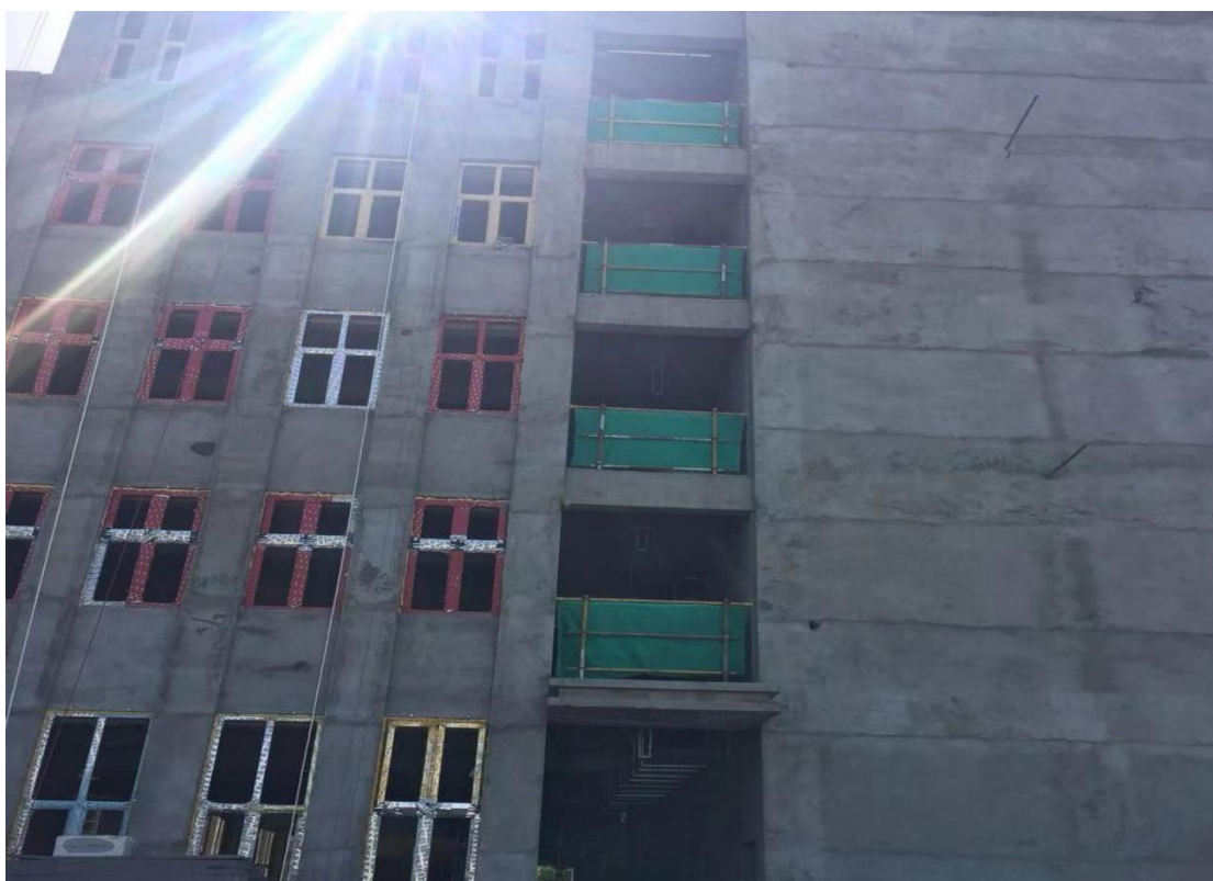
走廊两头洞口做双层防护并每层悬挂安全网
